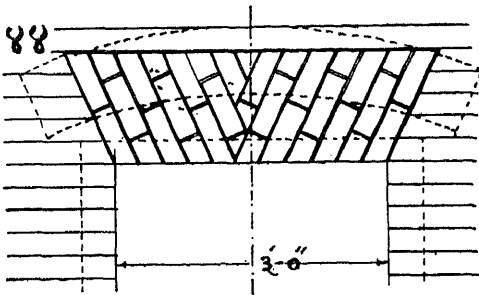
४४. French or Dutch arch : फ्रेंच-डच
